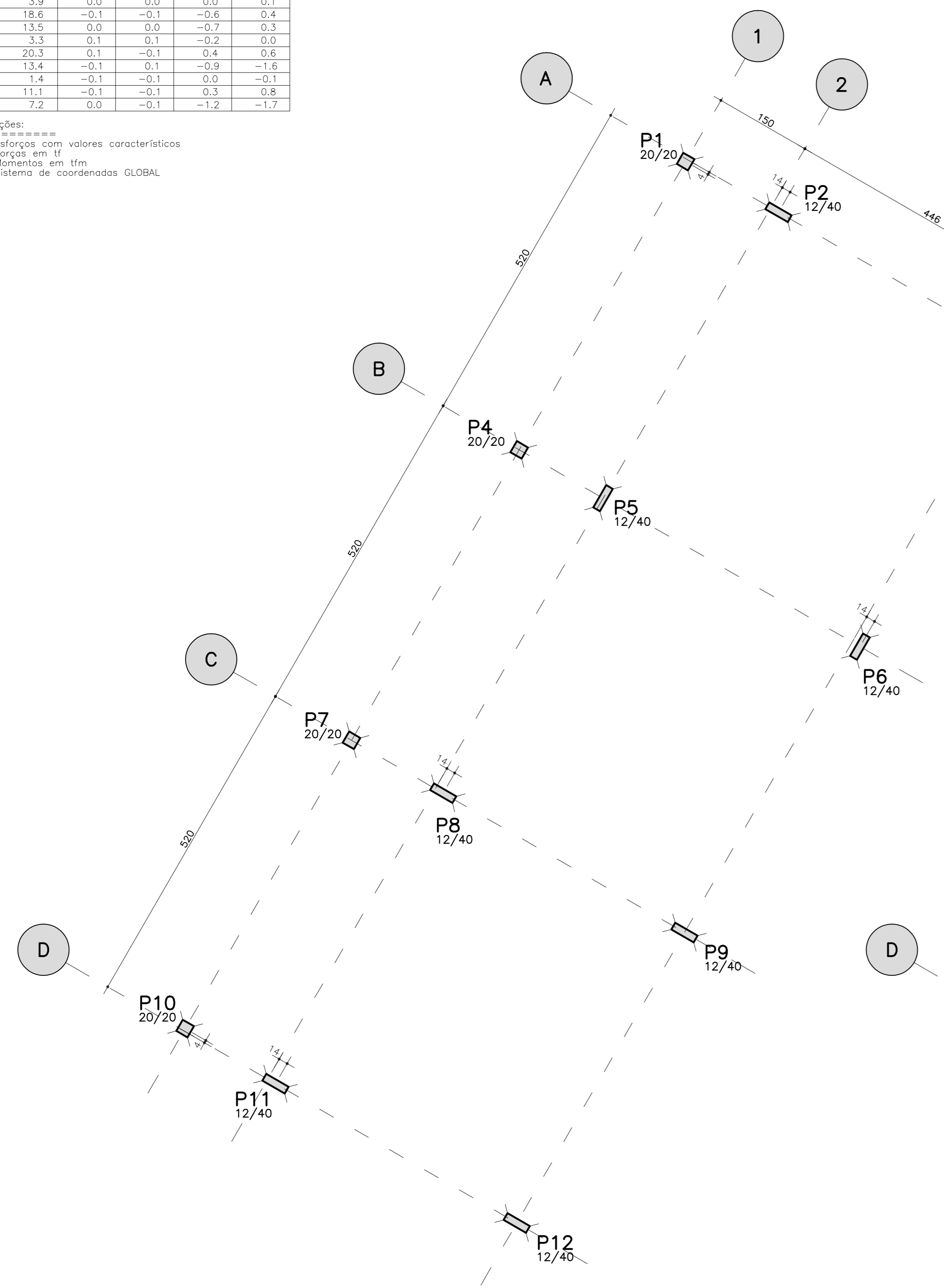
LOCALIZAÇÃO E CARGA DOS PILARES
