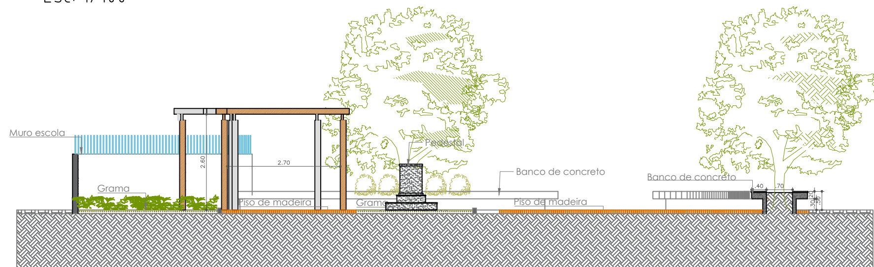
04 Corte AA Esc: 1/100
