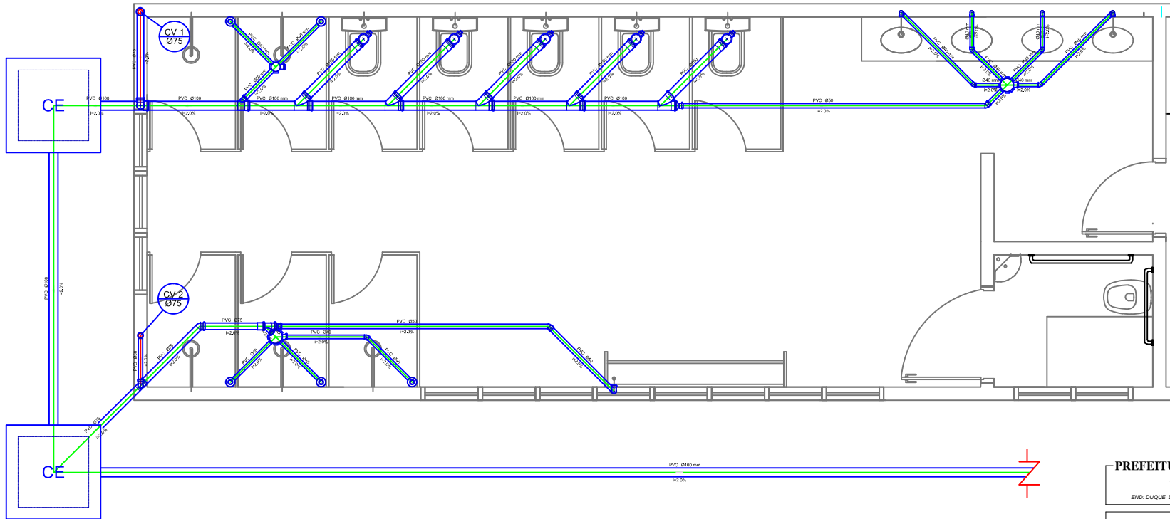
Detalhe S1 escala 1:20
