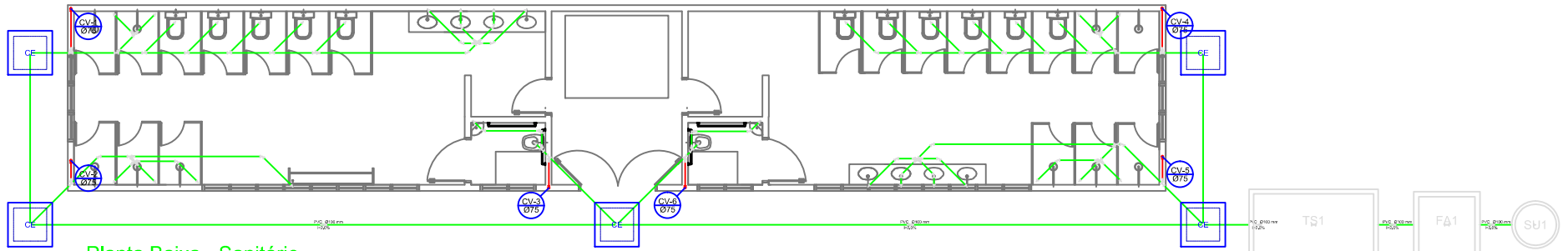
Planta Baixa - Sanitário escala 1:50
