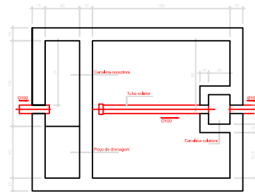
FILTRO ANAERÓBIO PLANTA BAIXA - ESC. 1:20
