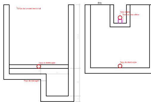
FILTRO ANAERÓBIO CORTES - ESC. 1:20
