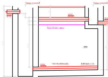
FILTRO ANAERÓBIO CORTE - ESC. 1:20
