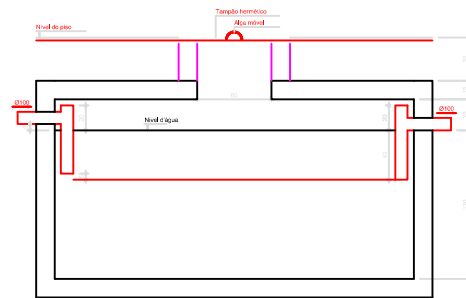
TANQUE SÉPTICO CORTE - ESC. 1:20
