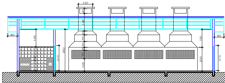
CORTE BB Esc. 1/50
