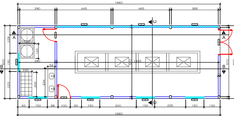
PLANTA BAIXA - MOQUEM ÁREA A EDIFICAR: 99,60M 2 Esc. 1/50
