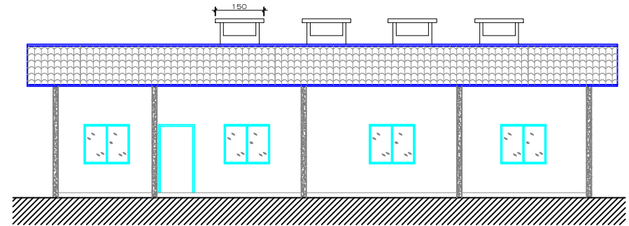
FACHADA Esc. 1/50
