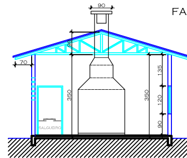
CORTE CC Esc. 1/50
