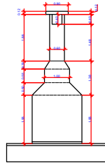
VISTA LATERAL ESCALA 1:50
