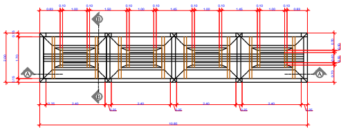
Detalhe ESCALA 1:50
