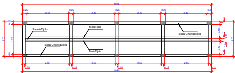
Detalhe ESCALA 1:50
