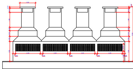
VISTA FRONTAL ESCALA 1:50
