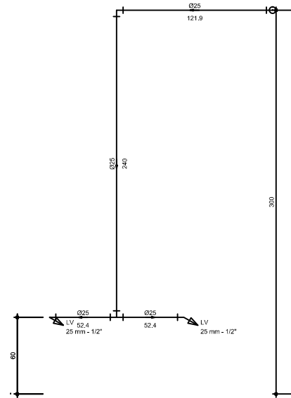
Vista 02 escala 1:25
